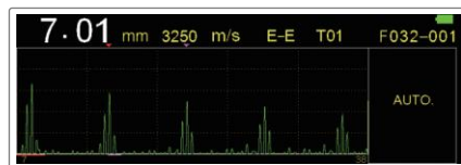
A-Scan
